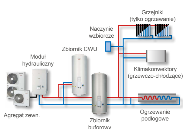
Ogrzewanie/chłodzenie 2-strefowe (wieloobiegowe) z produkcją CWU
