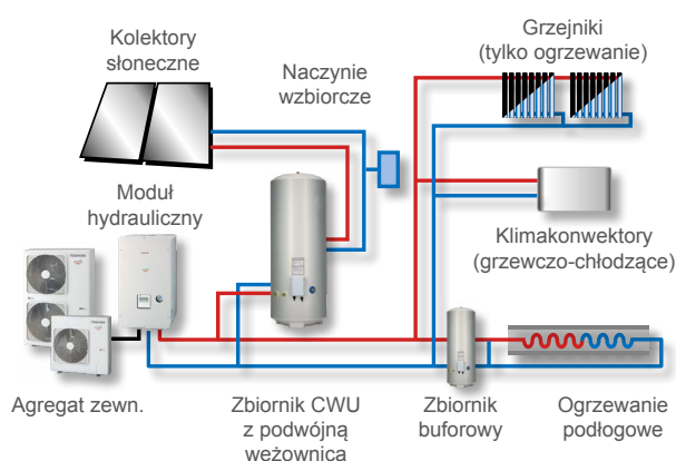
Ogrzewanie/chłodzenie 2-strefowe (wieloobiegowe) z produkcją CWU i panelami solarnymi
